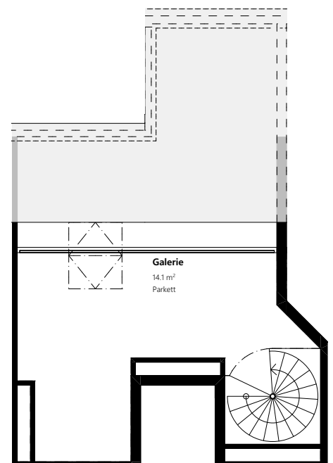
Galeriegeschoss
